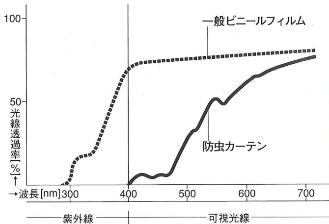
●一般ビニールフィルムとの光線透過率の比較
