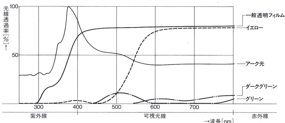
〈アキレスウェルディングカーテン〉光線透過グラフ
