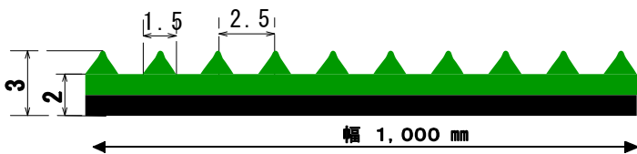
断面図
